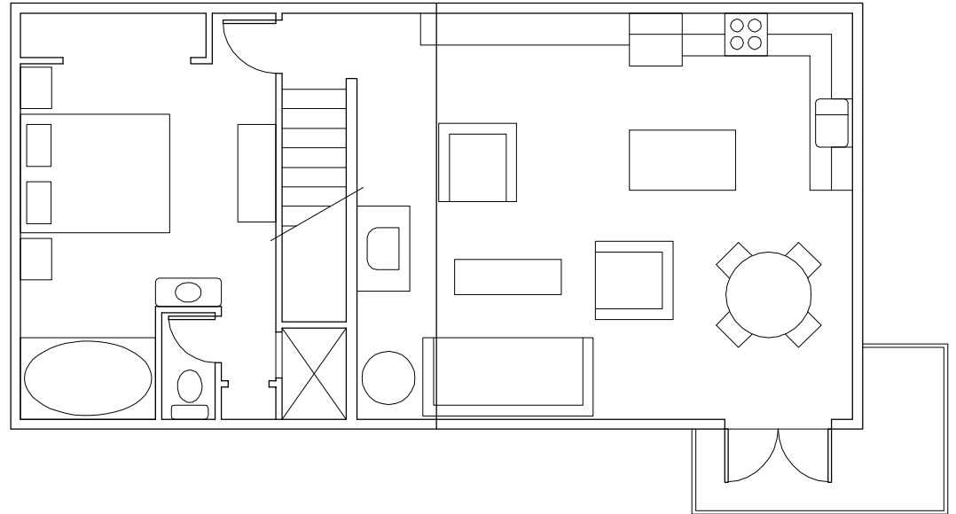
○ OPTION 2 SCALE: 1/8"=1'-0"
