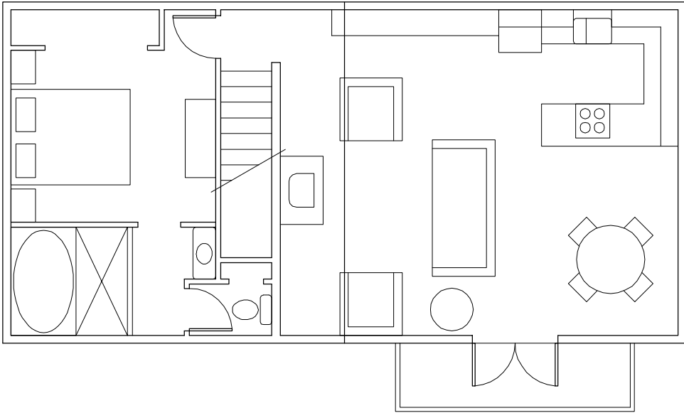
○ OPTION 1 SCALE: 1/8"=1'-0"
