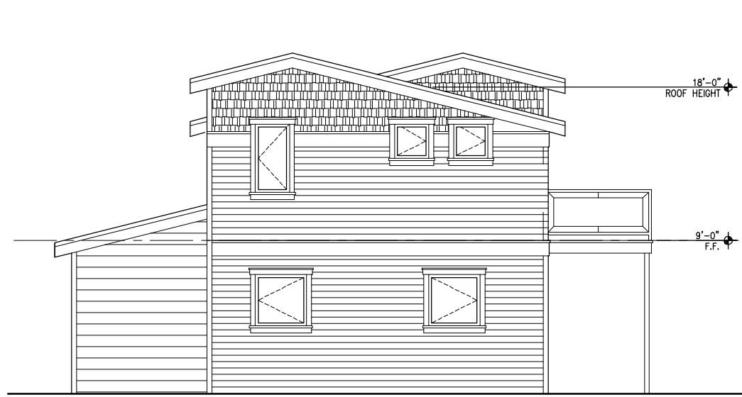
3 EAST ELEVATION A3.0 SCALE: 1/8"=1'-0"
