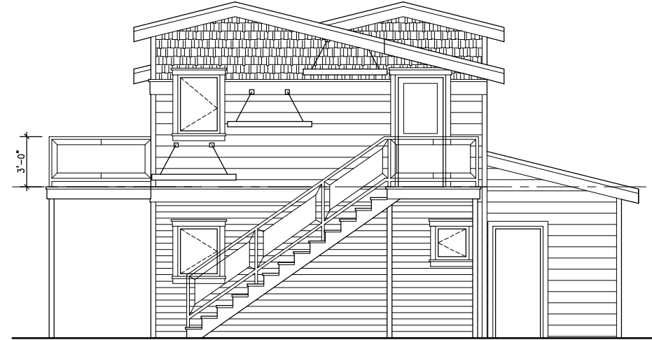
4 WEST ELEVATION A3.0 SCALE: 1/8"=1'-0"
